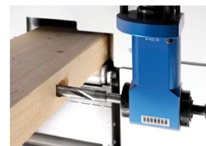
Wykonywanie otworów na czopty i kieszenie
