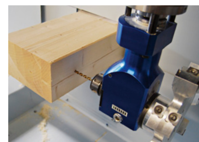
Wiercenie w poziomie
