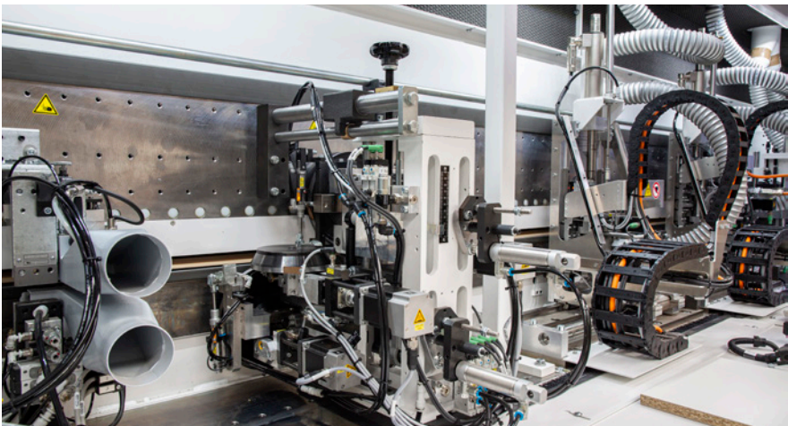
Racleur multiple MN11
