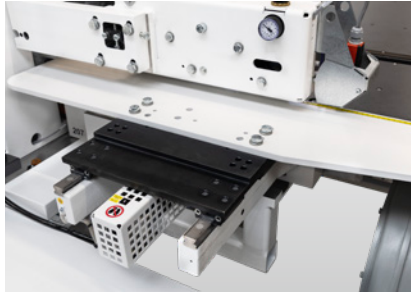
Réglage automatique du guide d'entrée
