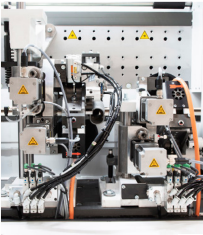
Agrégat de fraisage multi-étagé MS40
