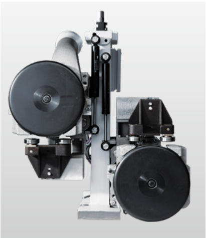
Agrégat de fraisage multiple MF21
