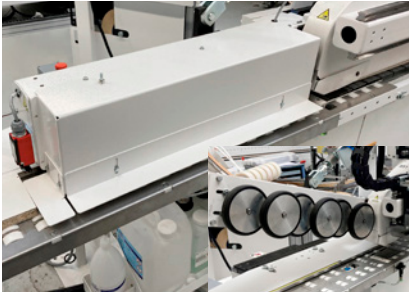
Dispositif d'introduction à 6 rouleaux
