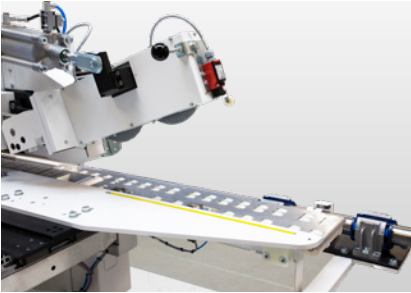
Dispositif d'introduction à 2 rouleaux
