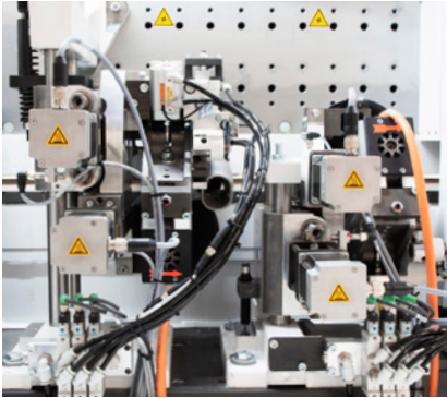
Agrégat de fraisage BF40 / MS40
