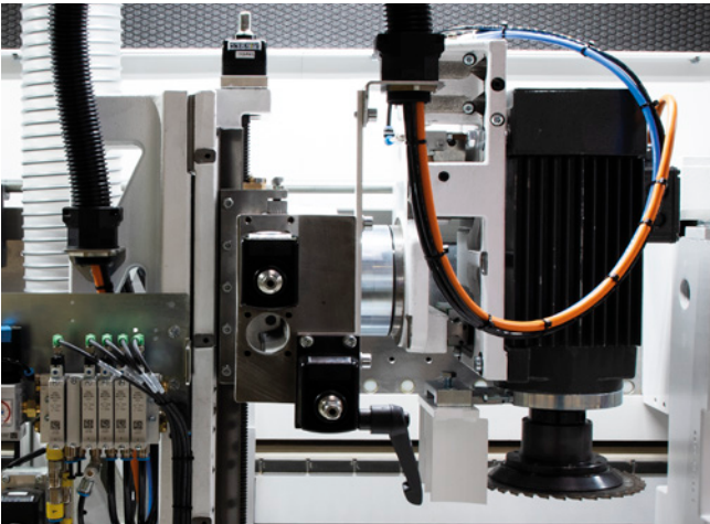
Agrégat de fraisage standard SF21
