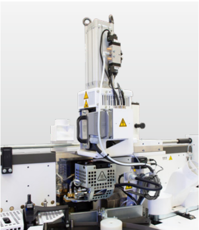
Unité d'encollage pour PUR
