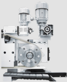
Presseur supérieur motorisé
