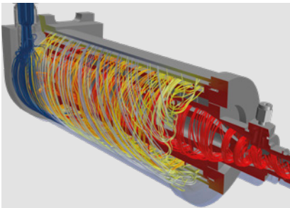
Ventilateur d'air chaud rotatif innovant
