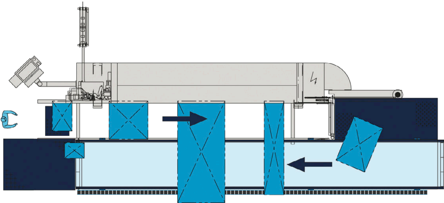
EDGETEQ S-500 avec retour de pièces LOOPTEQ
