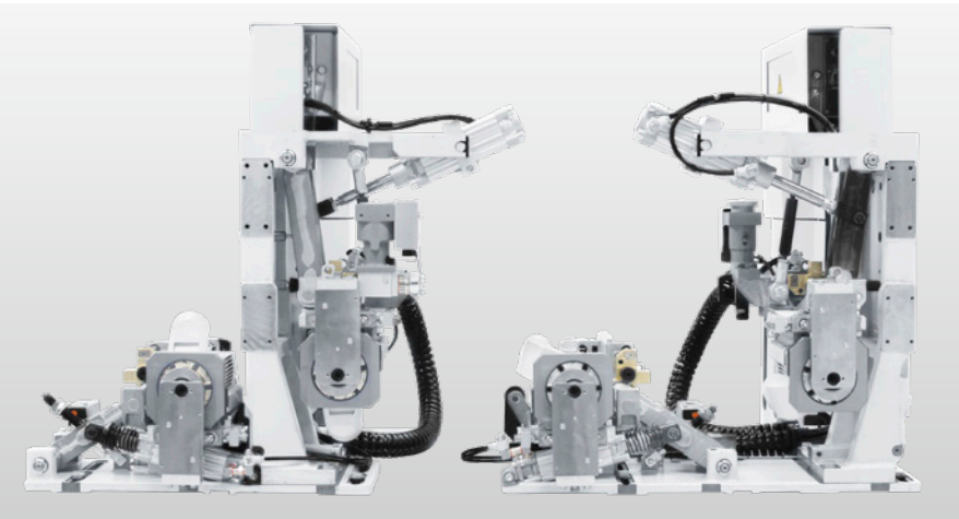
Agrégat de fraisage de forme FF32
