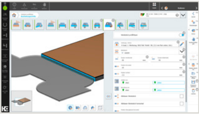
Simulation de pièce 3D avec trajectoire d'outil pouvant être affichée ou masquée.
