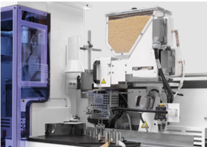
Agrégats d'encollage, application fiable de colle thermofusible
