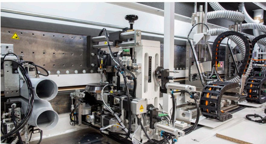
Multiziehklinge MN11
