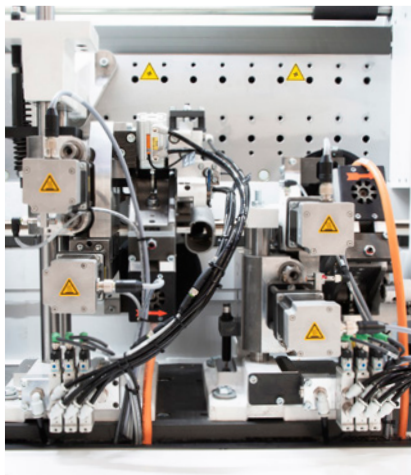
Mehrstufen Fräsaggregat MS40
