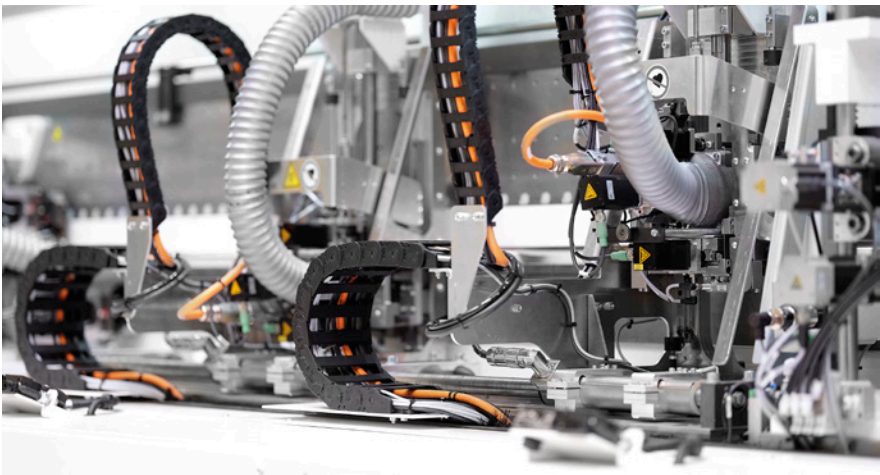
Multifunktions-Formfräsaggregat MF 60 Servotrim
