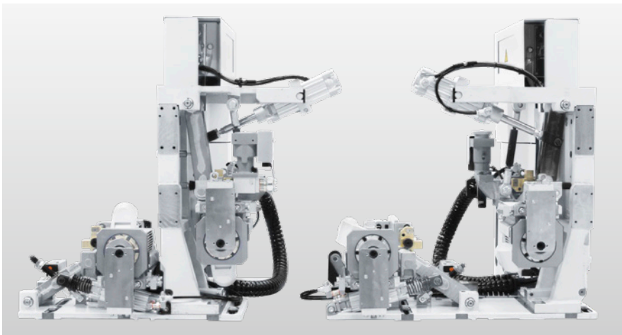
Formfräsaggregat FF32
